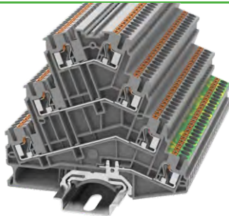
DS2.5-PE/3L
