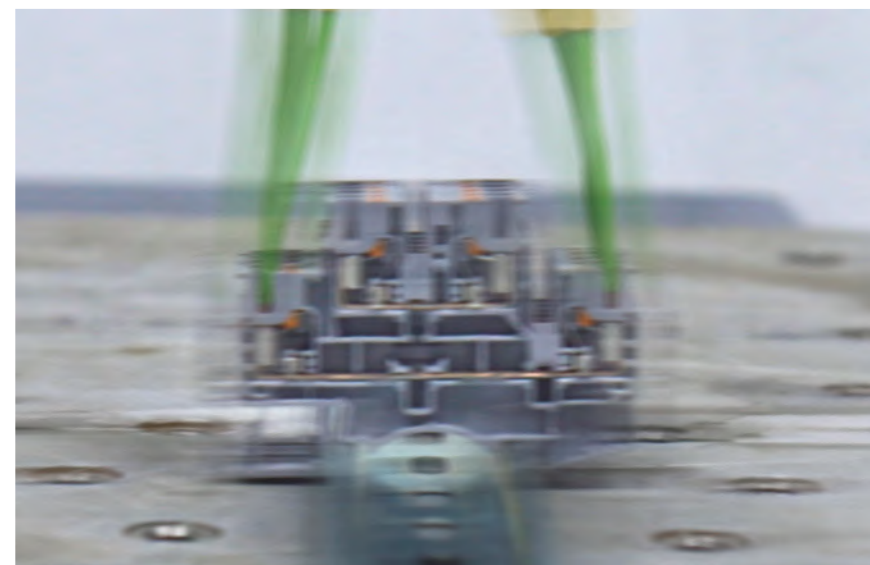
Испытания клемм на DIN-рейку на вибрационные нагрузки
