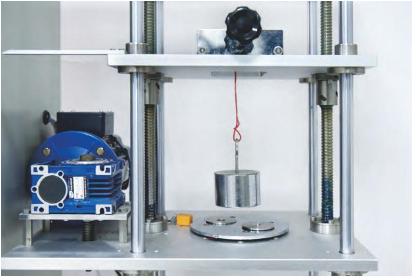
Испытание клемм на отрыв в зафиксированном положении
