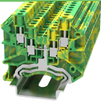
DC2.5-QU-PE
