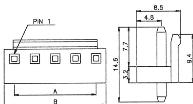
ВИЛКА ПРЯМАЯ
