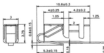
ВИЛКА УГЛОВАЯ
