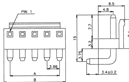
ВИЛКА УГЛОВАЯ
